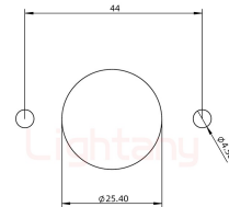
开孔尺寸
